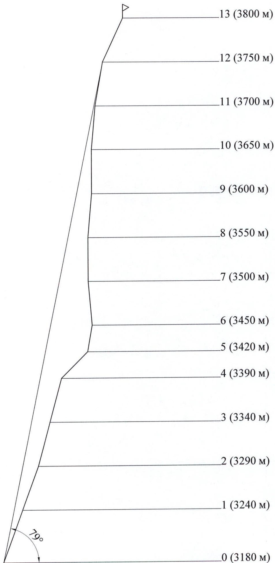
Профиль маршрута
