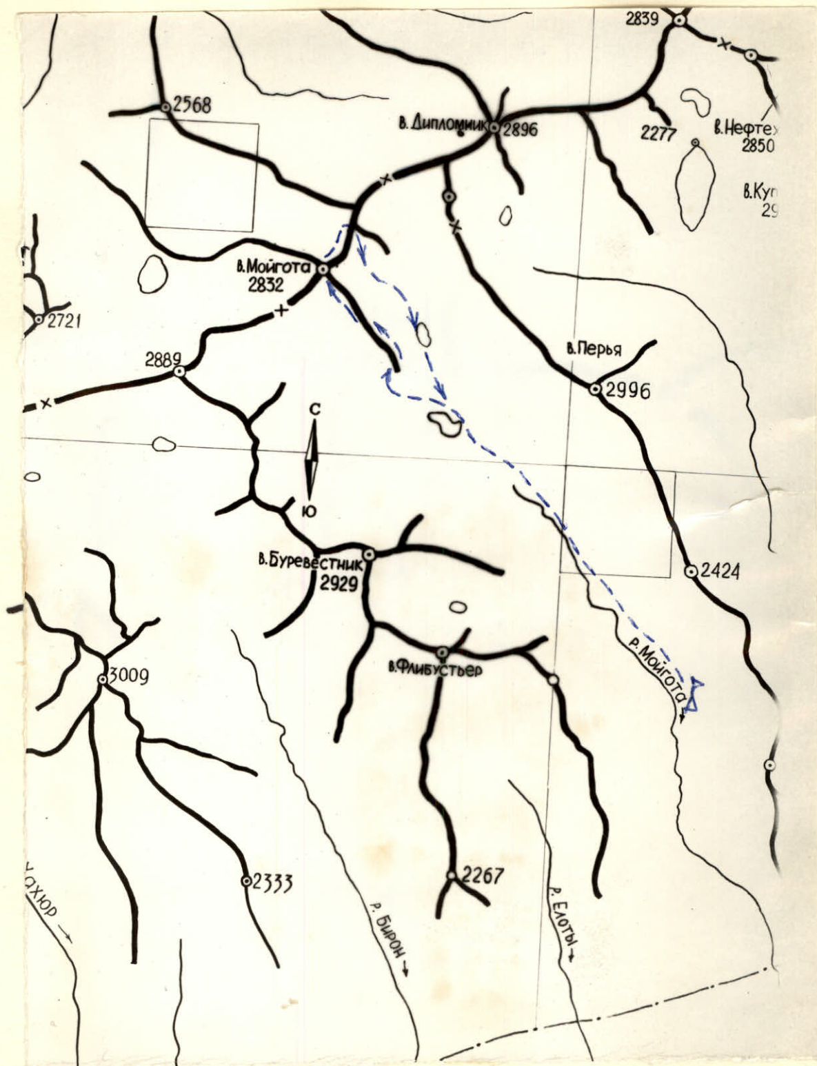
(карта -) Орографическая - схема цирка Мойготы
