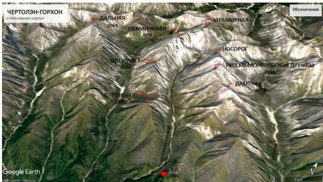
Фото 6. Схема вершин ущелья Чертолэн-Горхон
