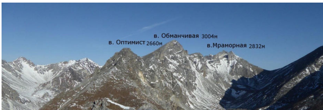
Фото 4. Фотопанорама верховья ущелья Чертолэн-Горхон с вершины Школьная
