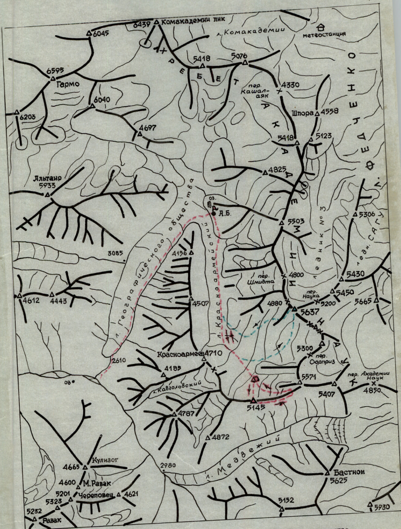
Рис.1 Карто-схема района ледников Географического общества и Красноармейский (Центральный Памир).
