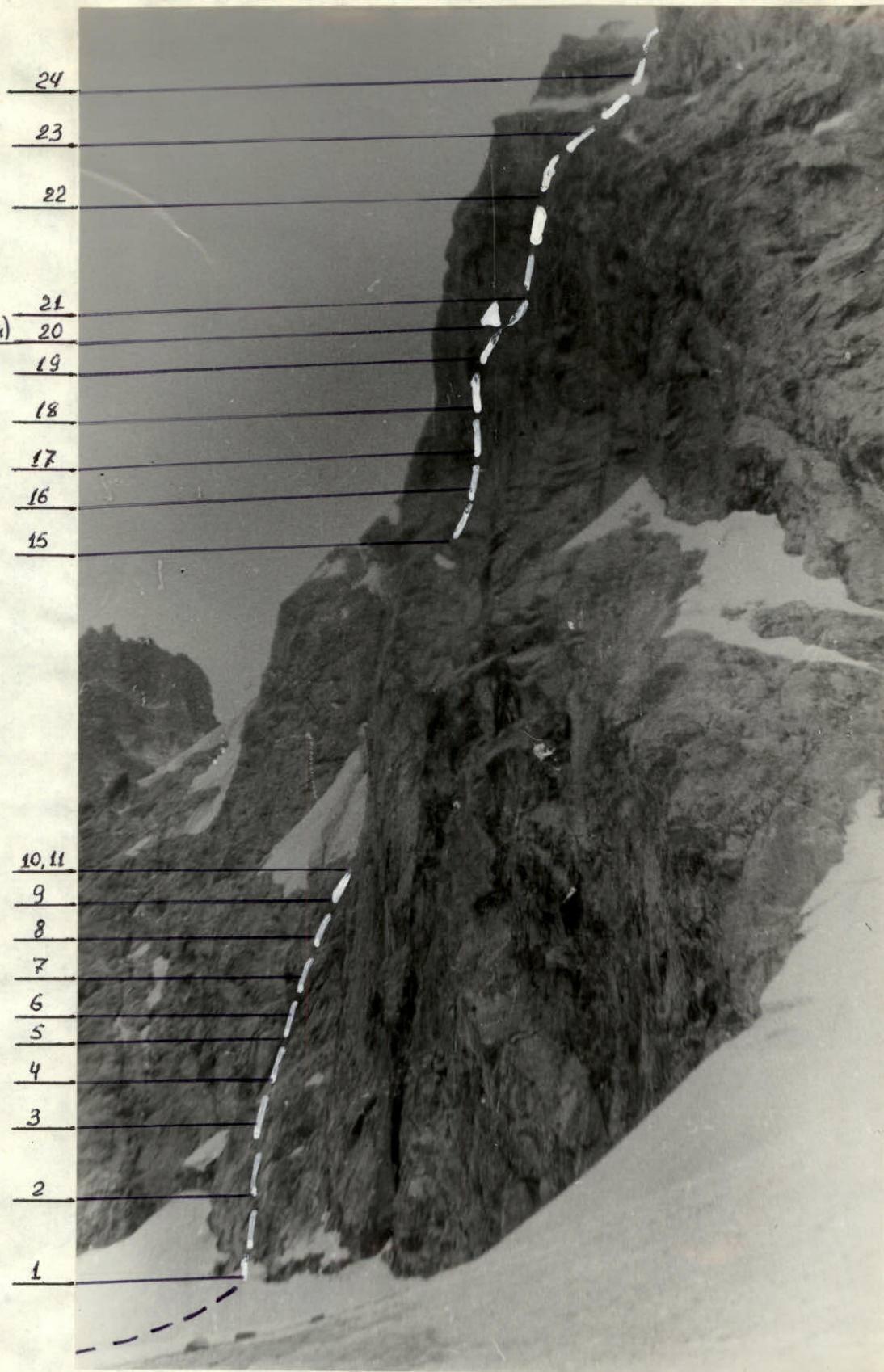
Профиль стены справа
