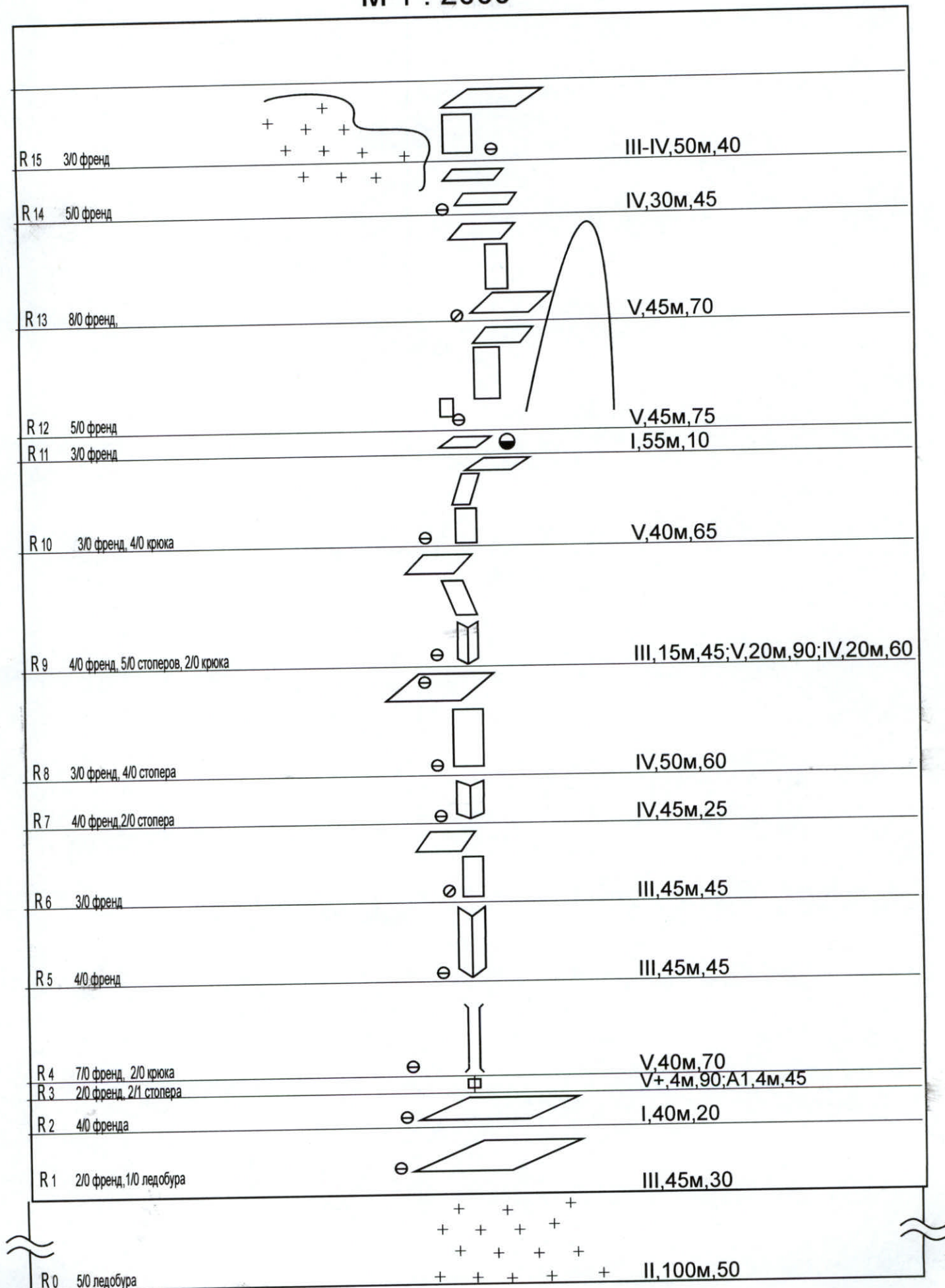
Рис.2.1 Схема в символах UIAA
