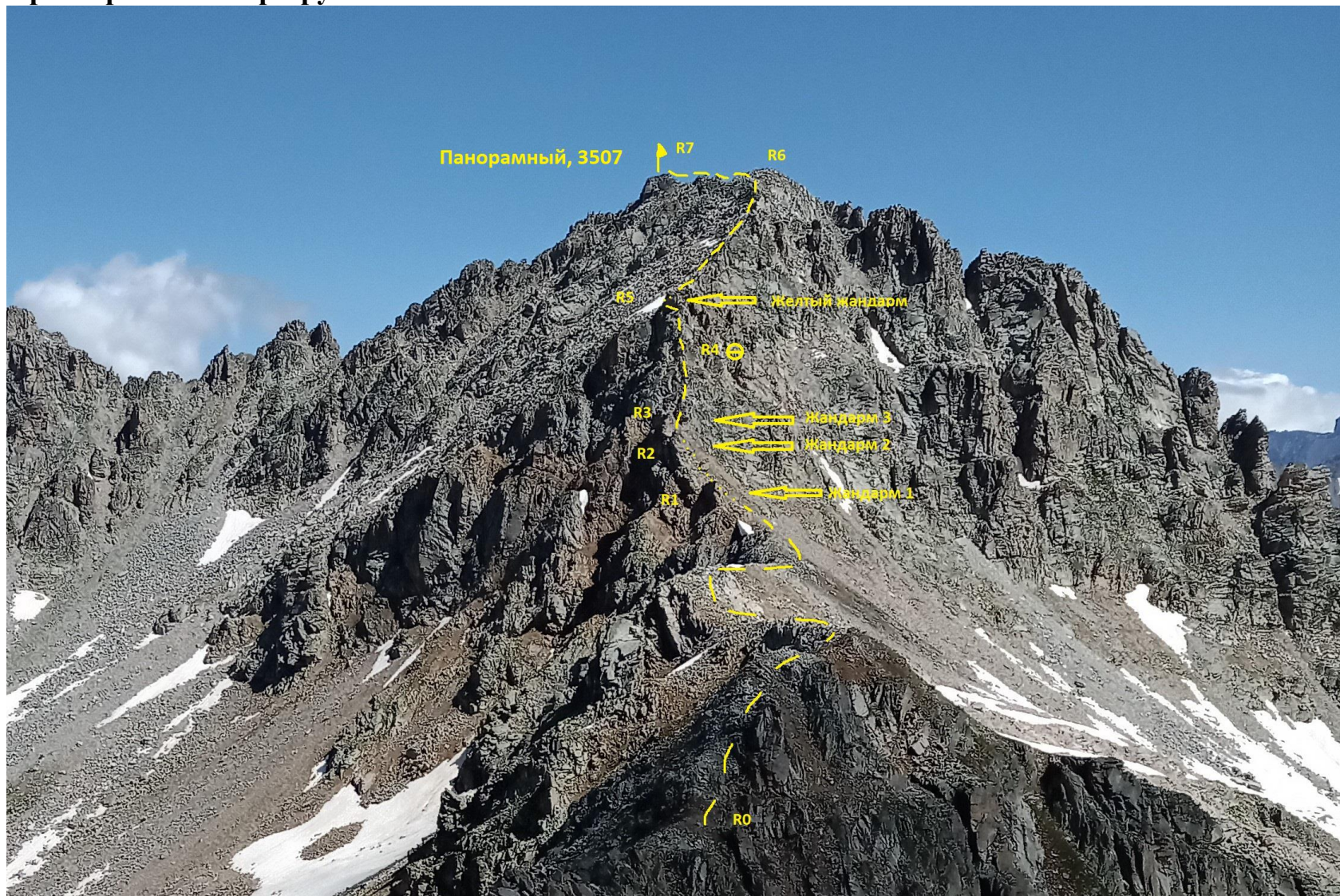
Фотография № 6. Техническая фотография маршрута (сделана 09.07.2021 со склона пика 3353).
