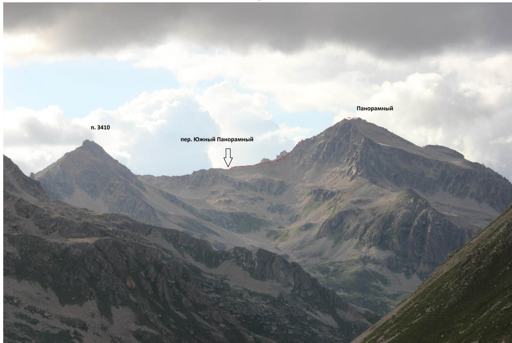
Фотография № 2. Профиль маршрута (сделана 30.07.2020 со склонов вершины Кичкинекольская башня).
